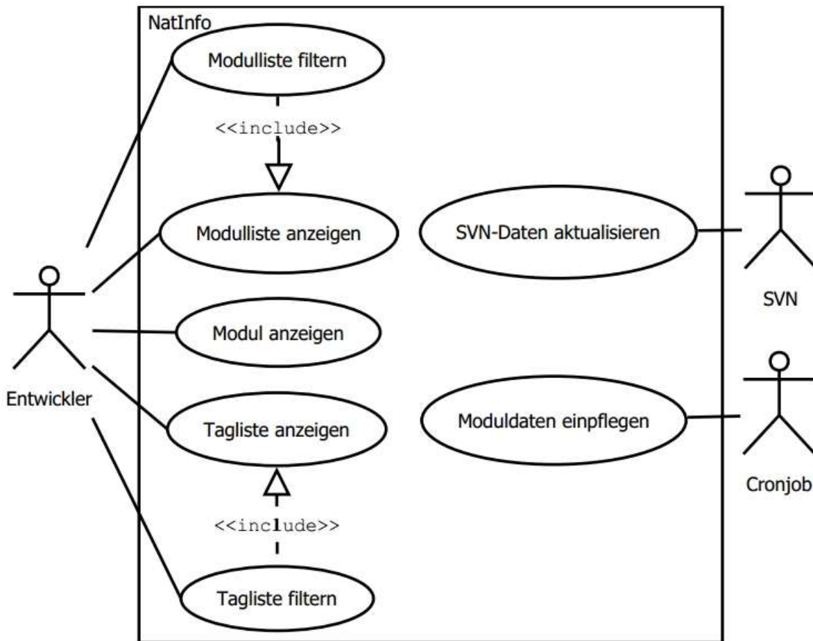
Abbildung 1: Use-Case-Diagramm
