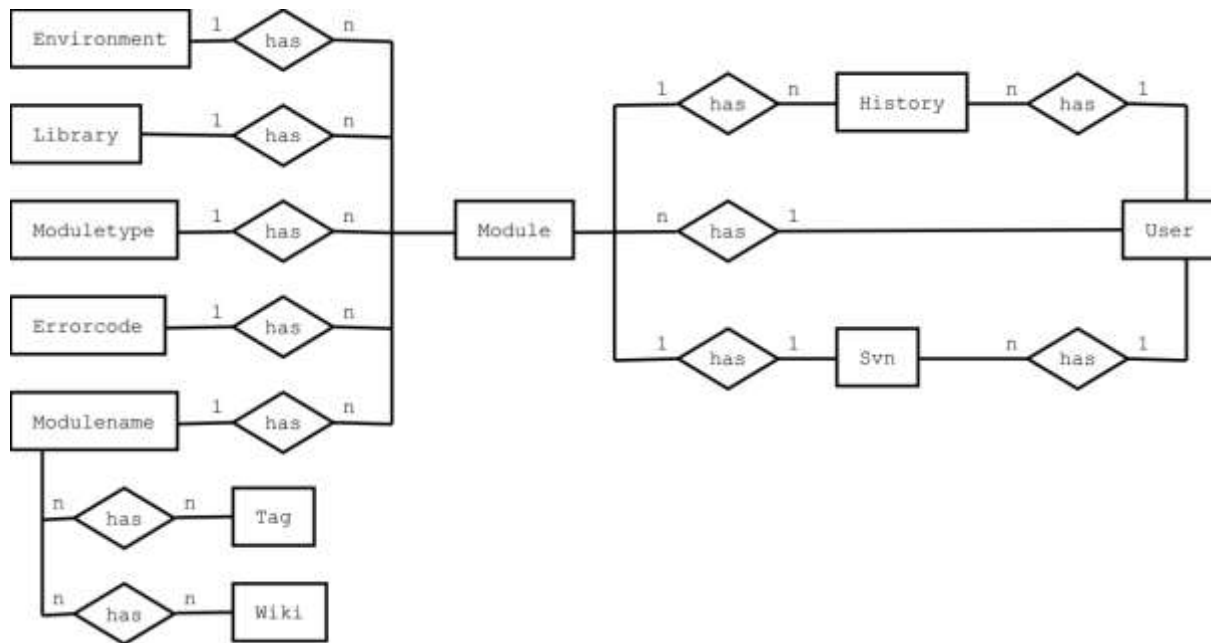
Abbildung 2: Entity-Relationship-Model
